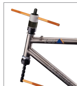
Voor balhoofdcups
