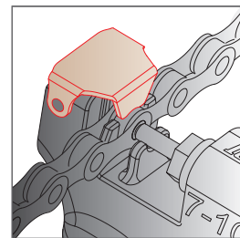
压链装置
