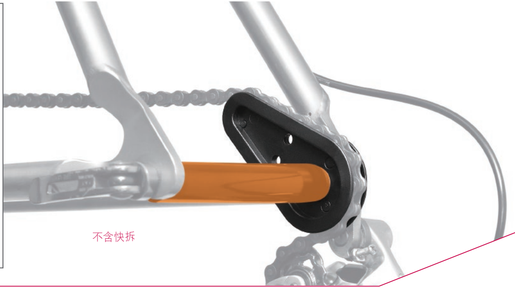
J 30C3 ChainMaster 贯穿轴用链条固定器 ■ 在运输车辆或维修后轮时，可以模拟工作状态来固定链条 ■ 适用于多种花鼓规格：142、146mm ■ 专利设计
